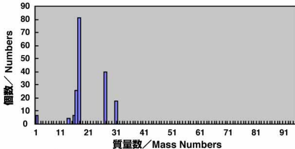
ETFEの高真空での発生ガスのマススペクトル Mass spectrum of out-gas from ETFE under full vacuum
